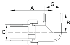
Соединение с полусгоном угловое в/в
